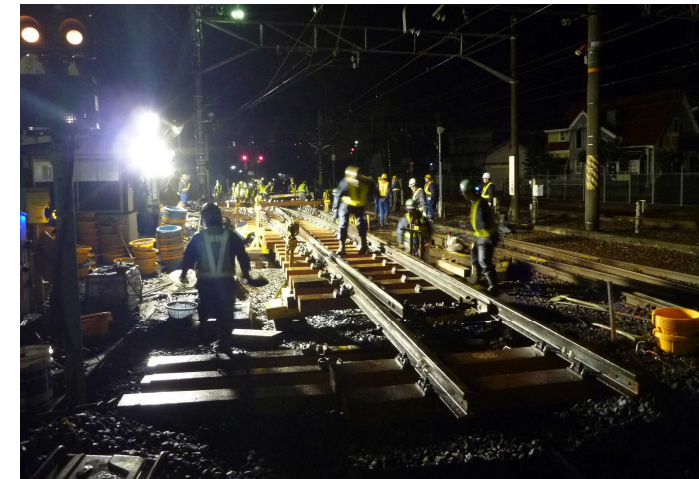
富田構内分岐器重軌条化工事
